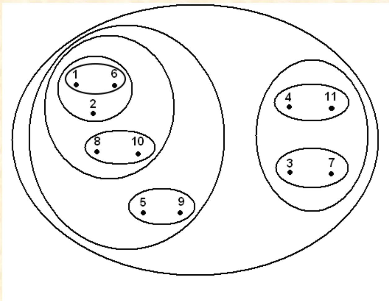
Slika 6.1. Venov dijagram
