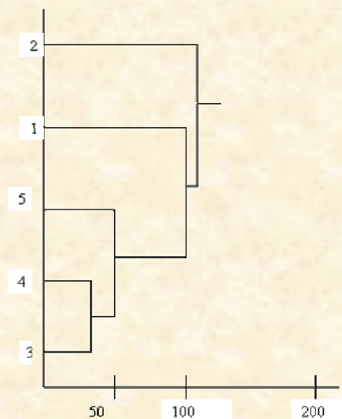
Slika 3. Dendrogram
